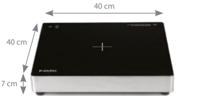
PODGRZEWACZ INDUKCYJNY IP WARM 4040 P157952 40 x 40 x 7 cm • 220-240 V • 1000 W • 50/60 Hz
