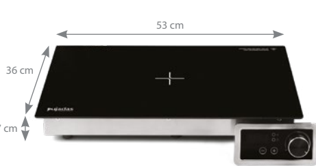
PODGRZEWACZ INDUKCYJNY DO WBUDOWANIA W BLAT IP WARM 5035 B P157951 53 x 36 x 7 cm • 220-240 V • 1000 W • 50/60 Hz • wymiar do wbudowania: 50 x 33 cm
