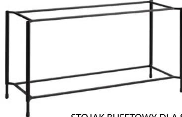
STOJAK BUFETOWY DLA SKRZYNEK GN 2/4 14029 57 x 21 x 28,5 cm Wielofunkcyjny stojak bufetowy składany wykonany z malowanego proszkowo metalu
